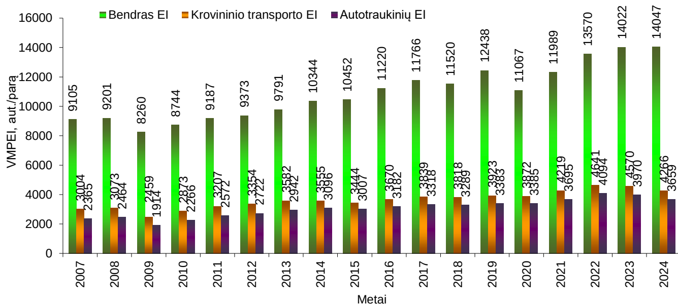
Vidutinio metinio paros eismo intensyvumo kitimas transporto koridoriuje Via Baltica nuo 2007-ųjų metų
