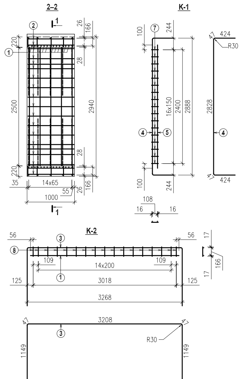
3,0 m angos pralaidos sekcijos SK-9 armavimas
