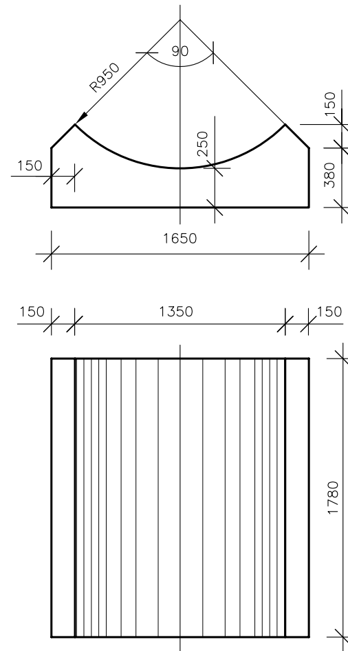
PAMATŲ BLOKAS PB-16
