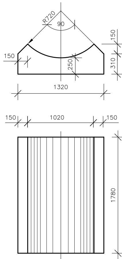
PAMATŲ BLOKAS PB-12
