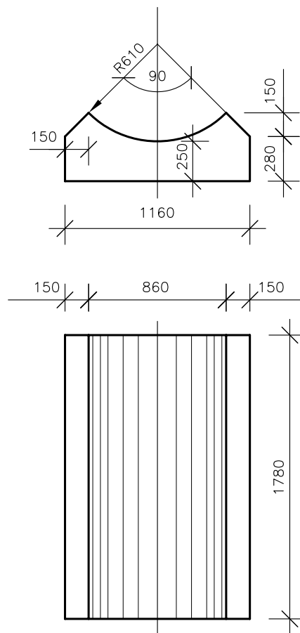
PAMATŲ BLOKAS PB-10
