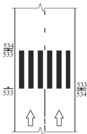
4 pav. Pėsčiųjų perėjos ženklinimo schema vienos eismo keliuose (gatvėse), turinčiose dvi ir daugiau eismo juostų
