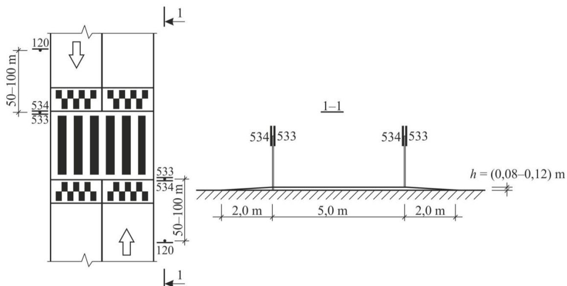
10 pav. Pėsčiųjų perėjos su trapecinės formos greičio mažinimo kalneliu ženklavimo schema dvipusio eismo keliuose (gatvėse)
