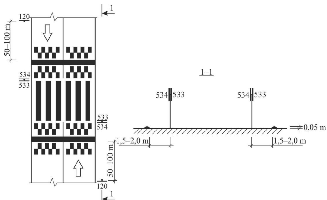
8 pav. Pėsčiųjų perėjos su apskritinės formos greičio mažinimo kalnėliu ženklinimo schema dvipusio eismo keliuose (gatvėse), kai leistinas greitis \leq 30 km/h
