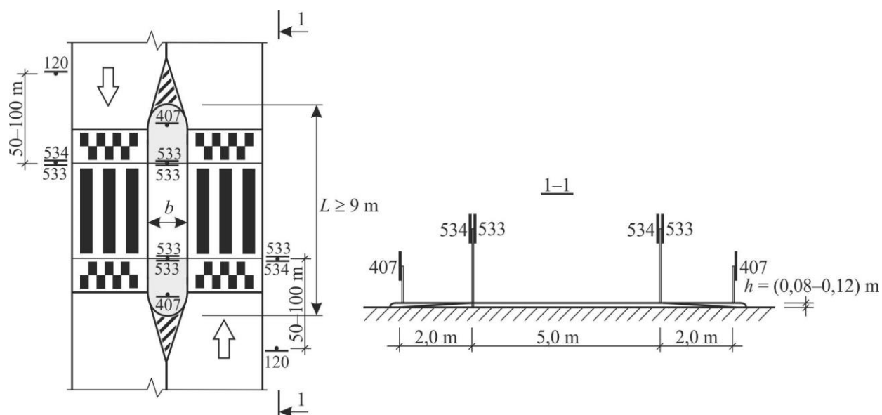
10 pav. Pėsčiųjų perėjos su trapecinės formos greičio mažinimo kalneliu ženklavimo schema dvipusio eismo keliuose (gatvėse)
