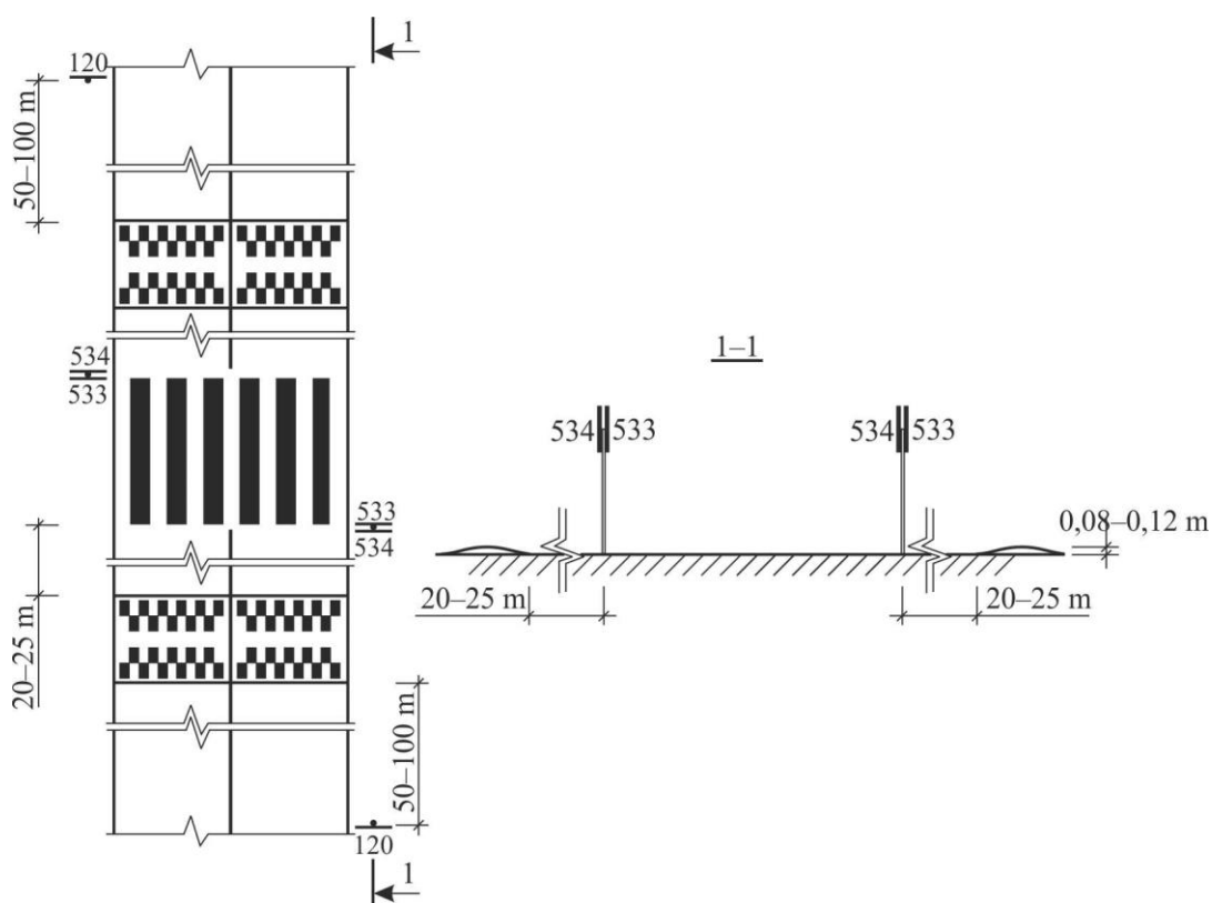
13 pav. Pėsčiųjų perėjos su sinusoidinės formos greičio mažinimo karneliu ženklavimo schema dvipusio eismo keliuose (gatvėse), kai leistinas greitis \leq 30 km/h
