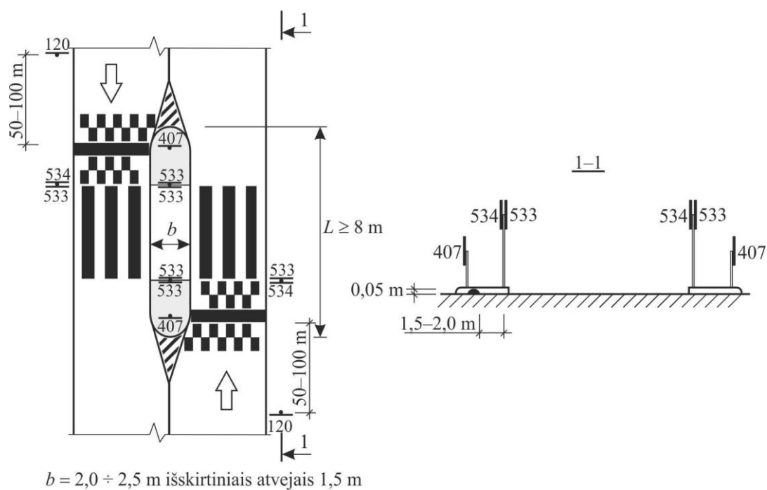
9 pav. Pėsčiųjų perėjos su apskritinės formos greičio mažinimo kalnėliu ir saugumo salele ženklinimo schema dvipusio eismo keliuose (gatvėse)
