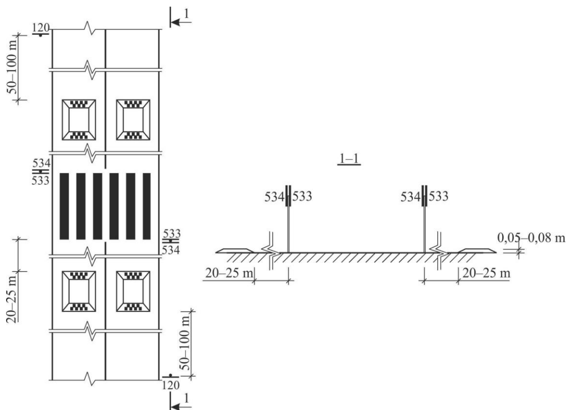
12 pav. Pėsčiųjų perėjos su daliniu trapezinės formos greičio mažinimo karneliu ženklavimo schema dvipusio eismo keliuose (gatvėse), kai leistinas greitis \leq 30 km/h
