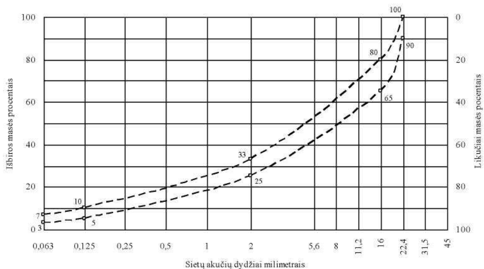
11 pav. Asfalto apatinio sluoksnio mišinys AC 22 AS
