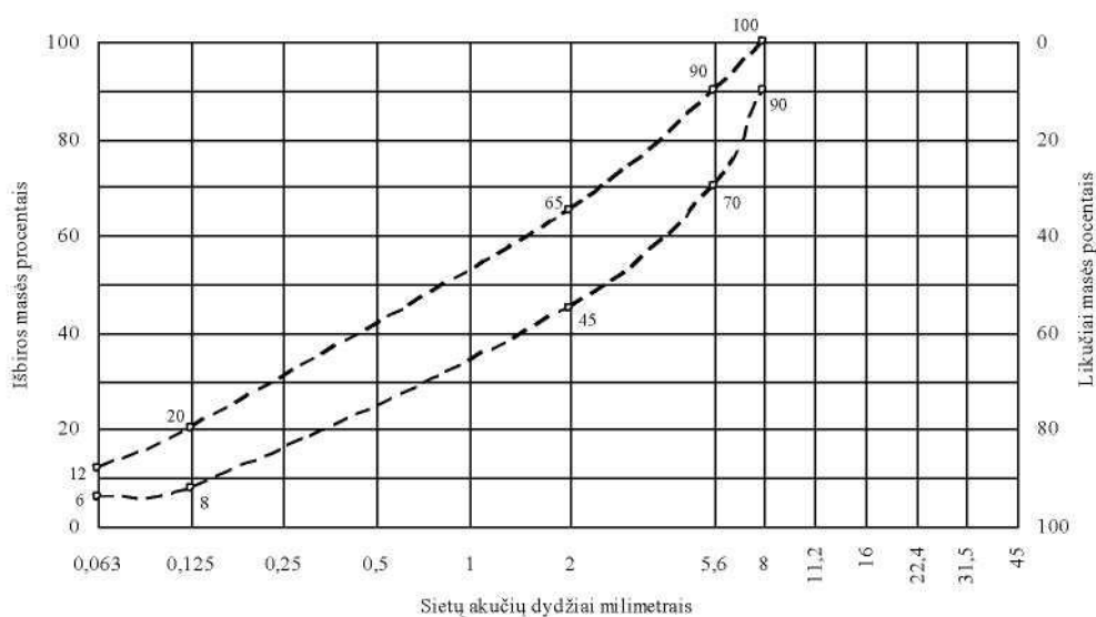
21 pav. Asfalto viršutinio sluoksnio asfaltbetonio mišinys AC 8 VL
