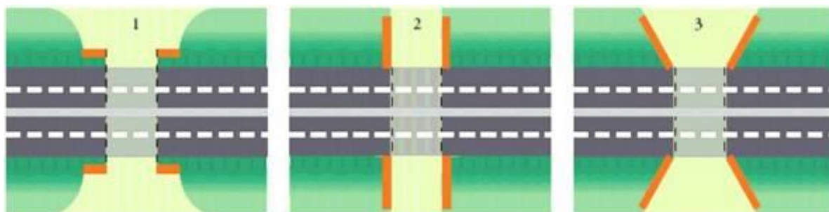
55 pav. Perėjos galų plokščių padėtis gali mažinti perėjos apšvietumą (2 priedas [21])
