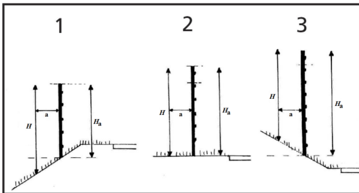
23 pav. Tvoros aukščio ( H_a ) skaičiavimas keliui esant ant sankasos (1), lygaus reljefo (2) ar iškastos (3). H – minimalus reikiamos tvoros aukštis; a – stambiesiems žinduoliams apie 50–75 cm
