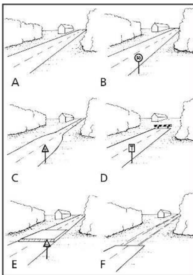
59 pav. Gyvūnų migravimo per kelią saugumo padidinimo priemonės. A – originali situacija; B – greičio mažinimas; C – greičio ir eismo intensyvumo mažinimas siaurinant kelią; D – visiškas eismo sustabdymas; E – greičio mažinimas papildomomis priemonėmis; F – visiškas kelio dangos pakeitimas į neatbaidančią gyvūnų (2 priedas [15])
